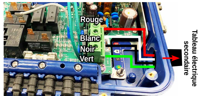
Boîtier de contrôle de 115/230 volts pour conversion sur le terrain
