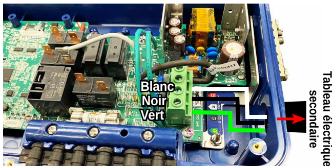
Boîtier de contrôle de 115 volts 30 ampères pour conversion sur le terrain
