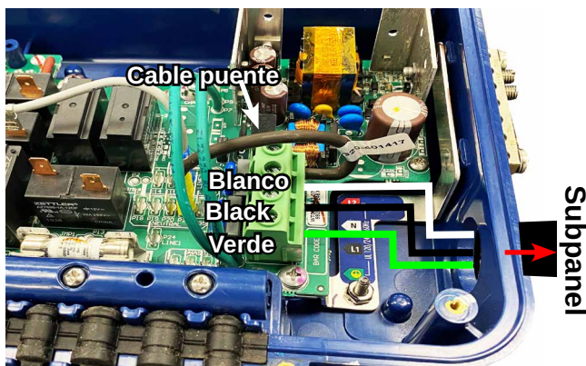
Caja de control de campo de conversión 115 V 30 A
