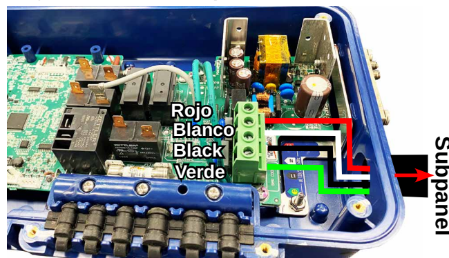
Caja de control de campo de conversión 115/230 V
